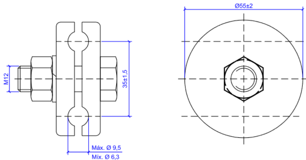
Figura 1 – Presilha tipo 1
