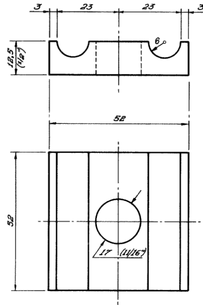
Figura 1 – Presilha tipo 1
